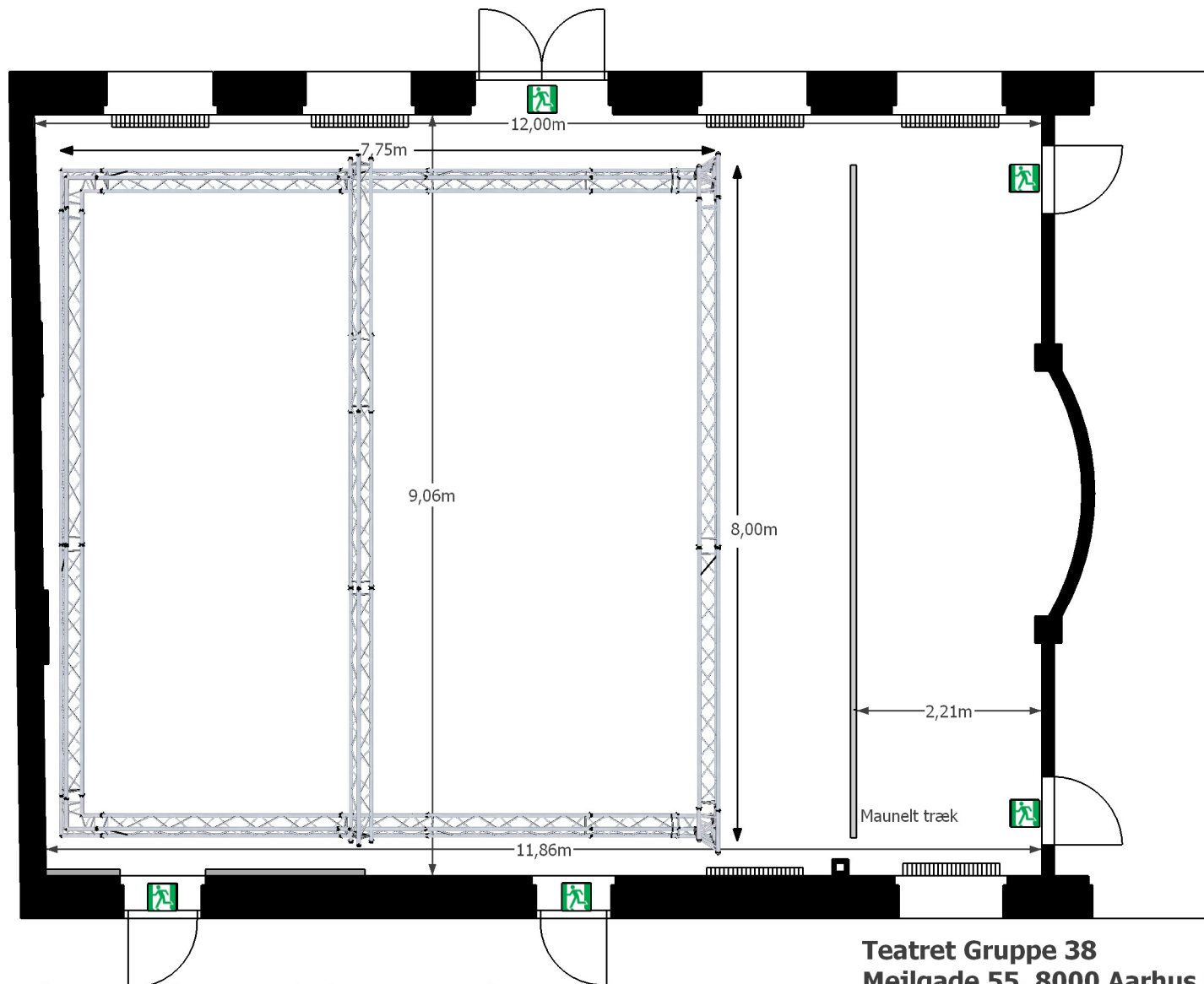
Plantegning med rig og træk
