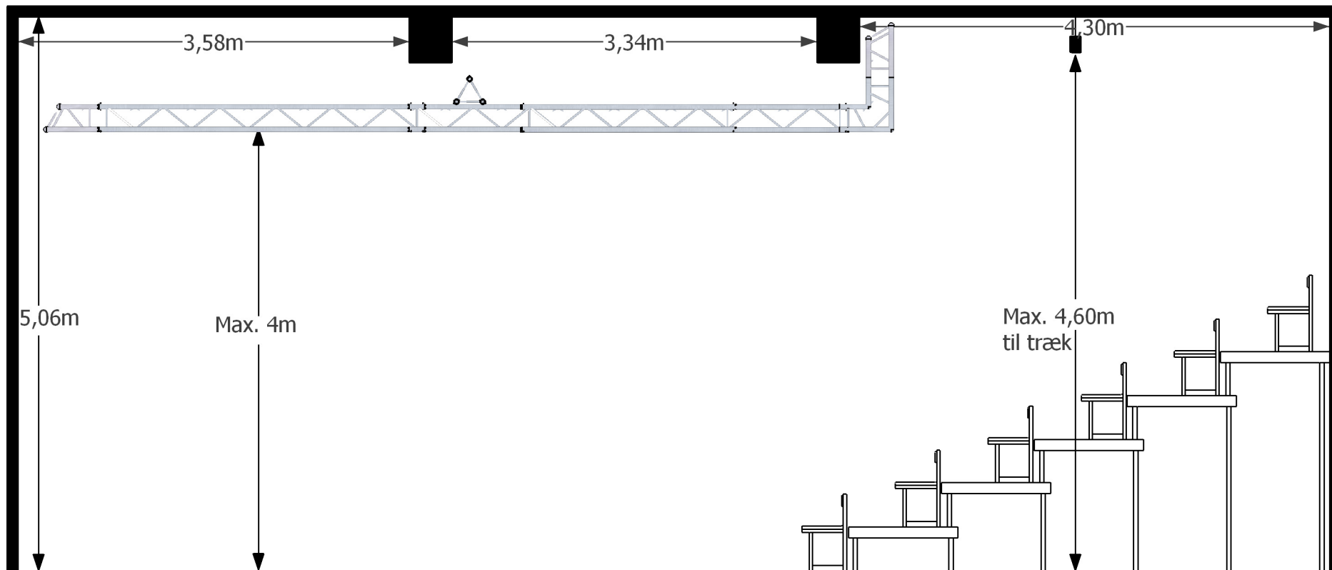
Snittegning teatersal
